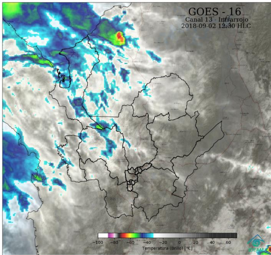
Nubosidad representada en la imagen satelital. Canal Infrarrojo - GOES 16 Septiembre 02 de 2018 - Hora 12:30 p.m.
